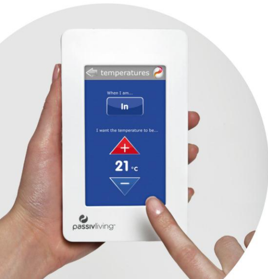
The PassivController
